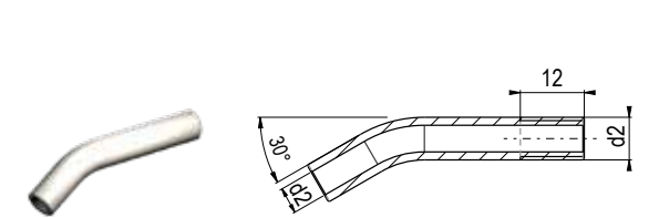
Prolunga per ugello di refrigerazione Cooling nozzle extensions
