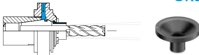
DISCHETTO PER REFRIGERAZIONE - FLUSH DISK
